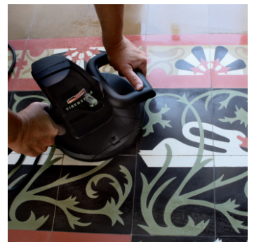
Verwendung einer Handmaschine 8"
